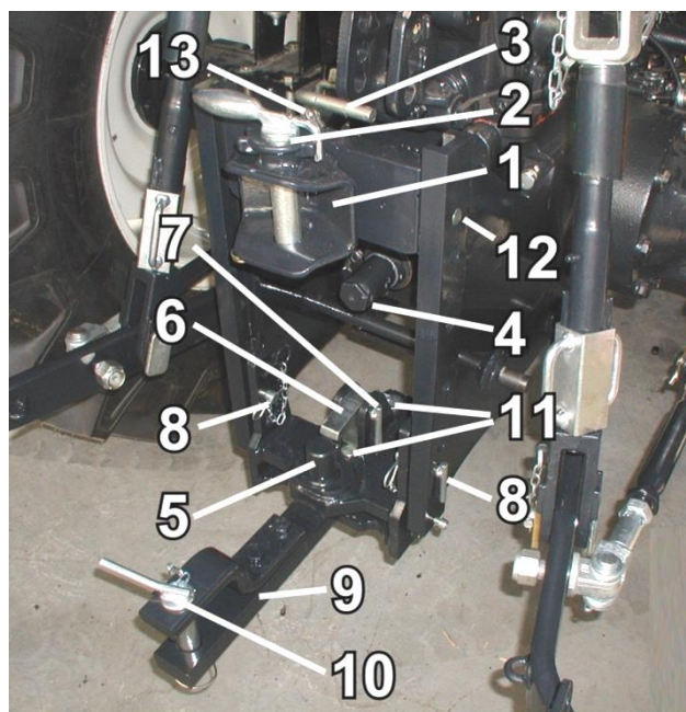
Rys. 4.6.2. Zaczepy
