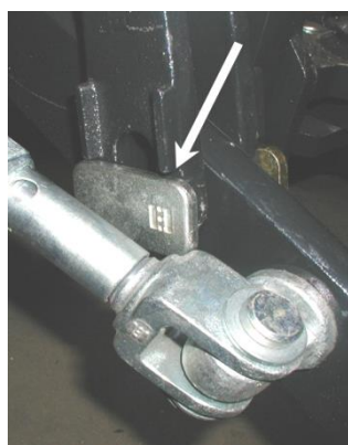
Rys. 4.6.3. Mocowanie wieszaków do cięgieł dolnych nieprzesuwnie - łeb i podkładka sworznia ustawione poziomo
