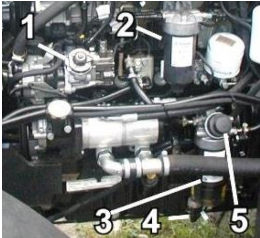
Rys. 5.3.4. Układ zasilania paliwem 1-pompa wtryskowa, 2- filtr paliwa, 3- separator, 4- korek spustowy, 5- ręczna pompa podająca.
