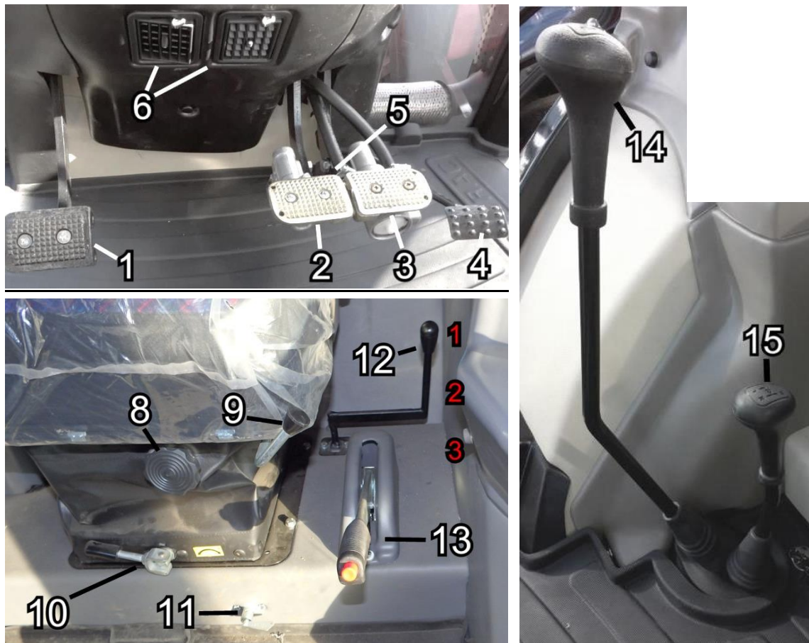
Rys. 3.4. Dźwignie sterowania ciągnikiem - opis w tekście
