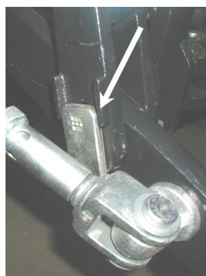
Rys. 4.6.4. Mocowanie wieszaków do cięgieł dolnych przesuwnie - łeb i podkładka sworznia ustawione pionowo
