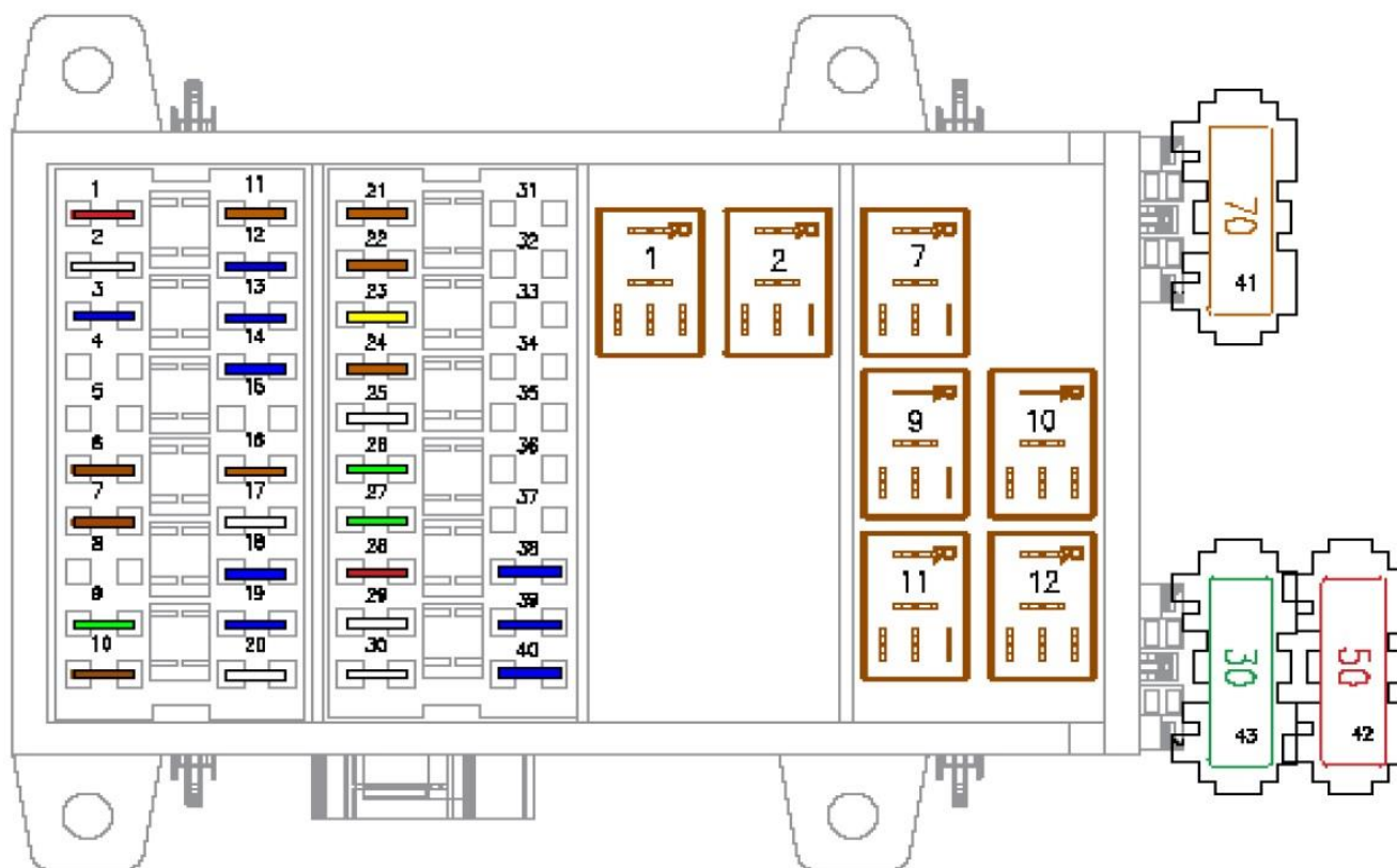
Rys. 5.4.3 Rozmieszczenie bezpieczników i przekaźników w skrzynce bezpieczników.
