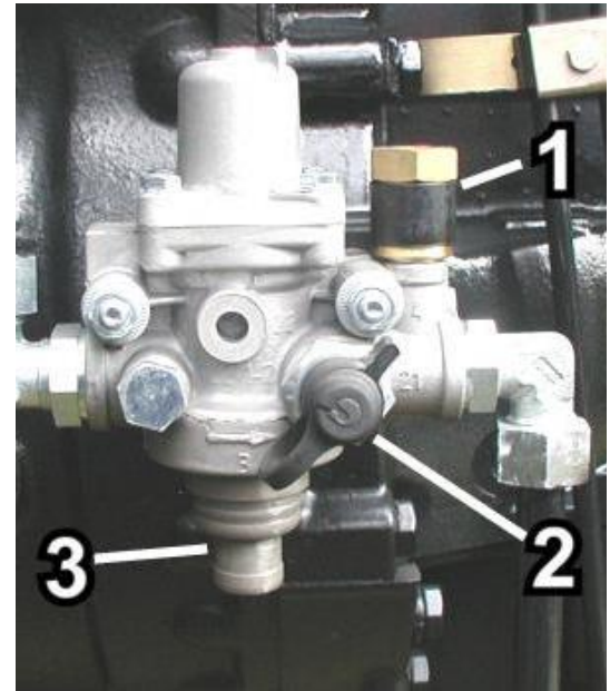
Rys. 5.15. Regulator ciśnienia
