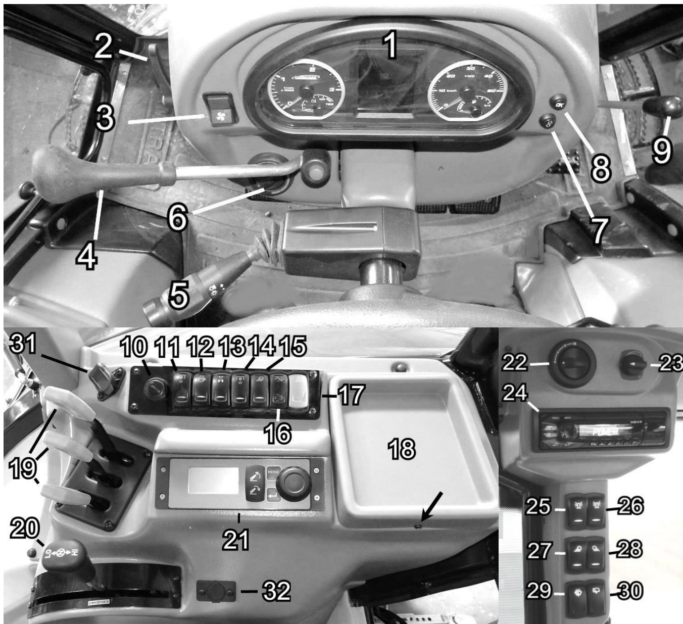
Rys. 3.1 Tablica rozdzielcza - opis w tekście.
