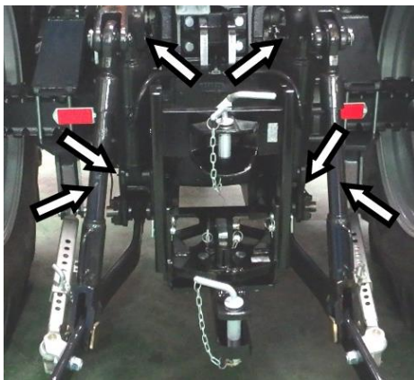
Rys. 5.9.5. Punkty smarowania sworzni siłowników TUZ
