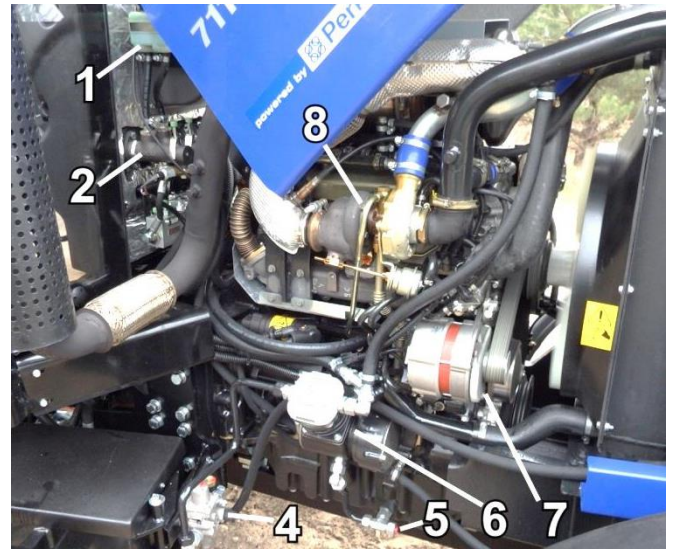
Rys. 5.3.3. Prawa strona silnika.
