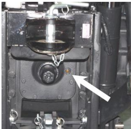
Rys. 5.9.4. Wziernik kontrolny poziomu oleju w układzie napędowym
