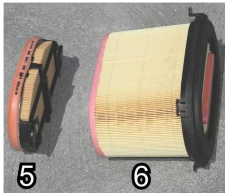
Rys. 5.3.6. Filtr powietrza 1-obudowa, 2- pokrywa, 3- zbiorniczek pyłu, 4 - zamki mocowania pokrywy, 5- wkład wstępny, 6- wkład dokładnego oczyszczenia.
