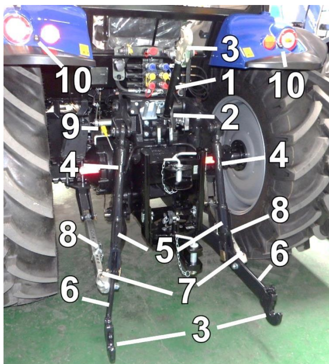
Rys. 4.6.1. Trzypunktowy układ zawieszenia (TUZ)
