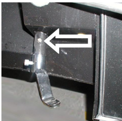
Rys. 5.8.1. Punkt smarowania tulei kolumny rewersu
