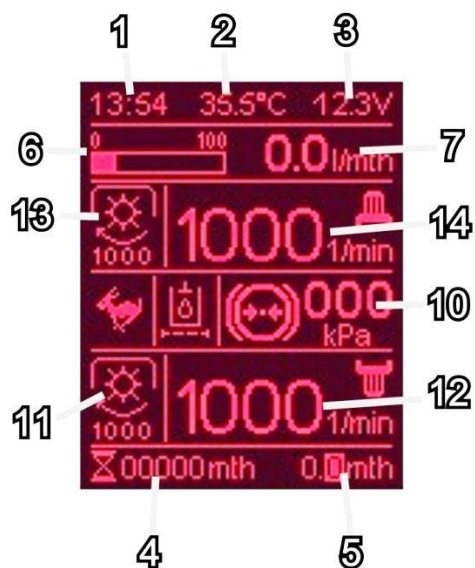
Rys. 3.3 Wyświetlacz centralny LCD.
