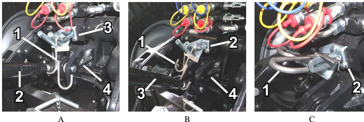
Rys. 4.6.5. Podwieszanie cięgła dolnego na wieszaku
